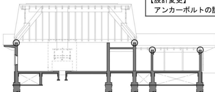
【南側断面図】
