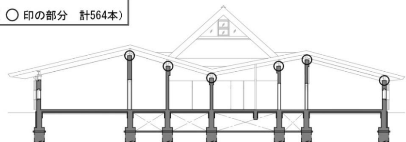
【東側断面図】
