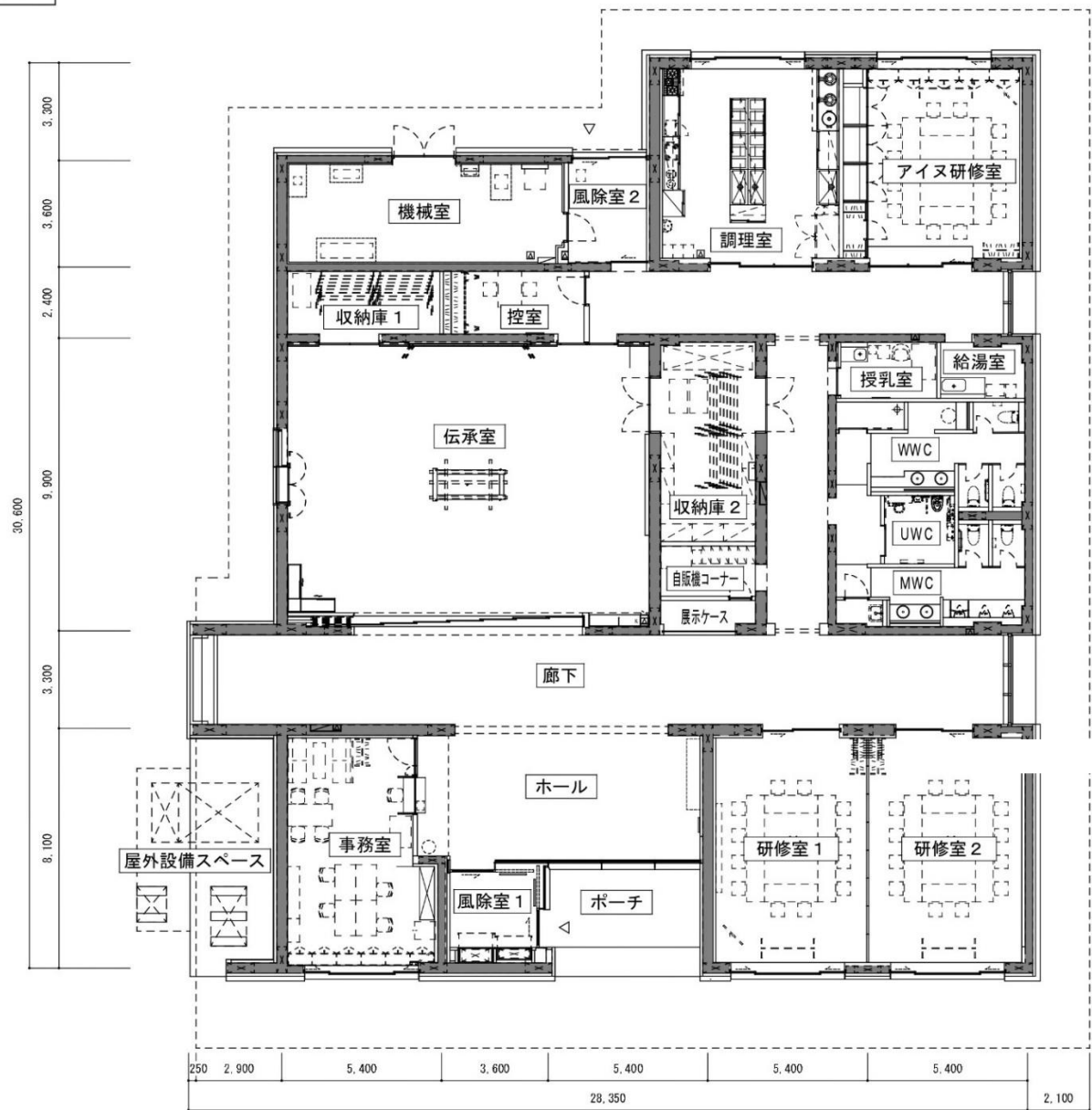
平面図
