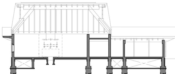
【南側断面図】
