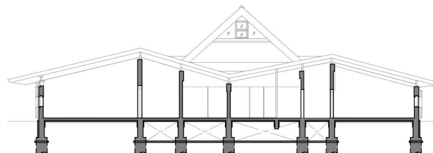
【東側断面図】
