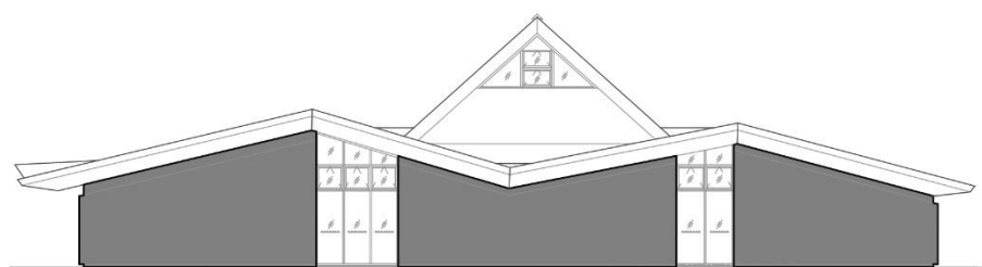
【東側立面図】
