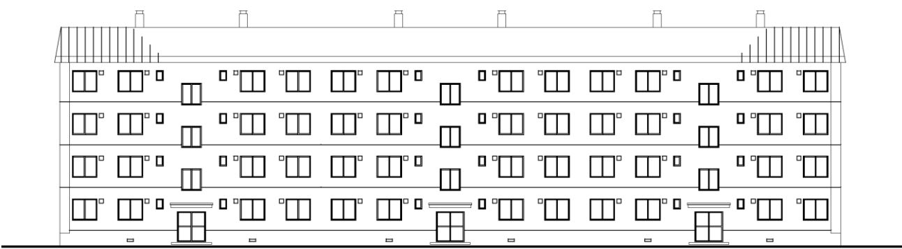
北側立面図
