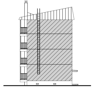
東側立面図
