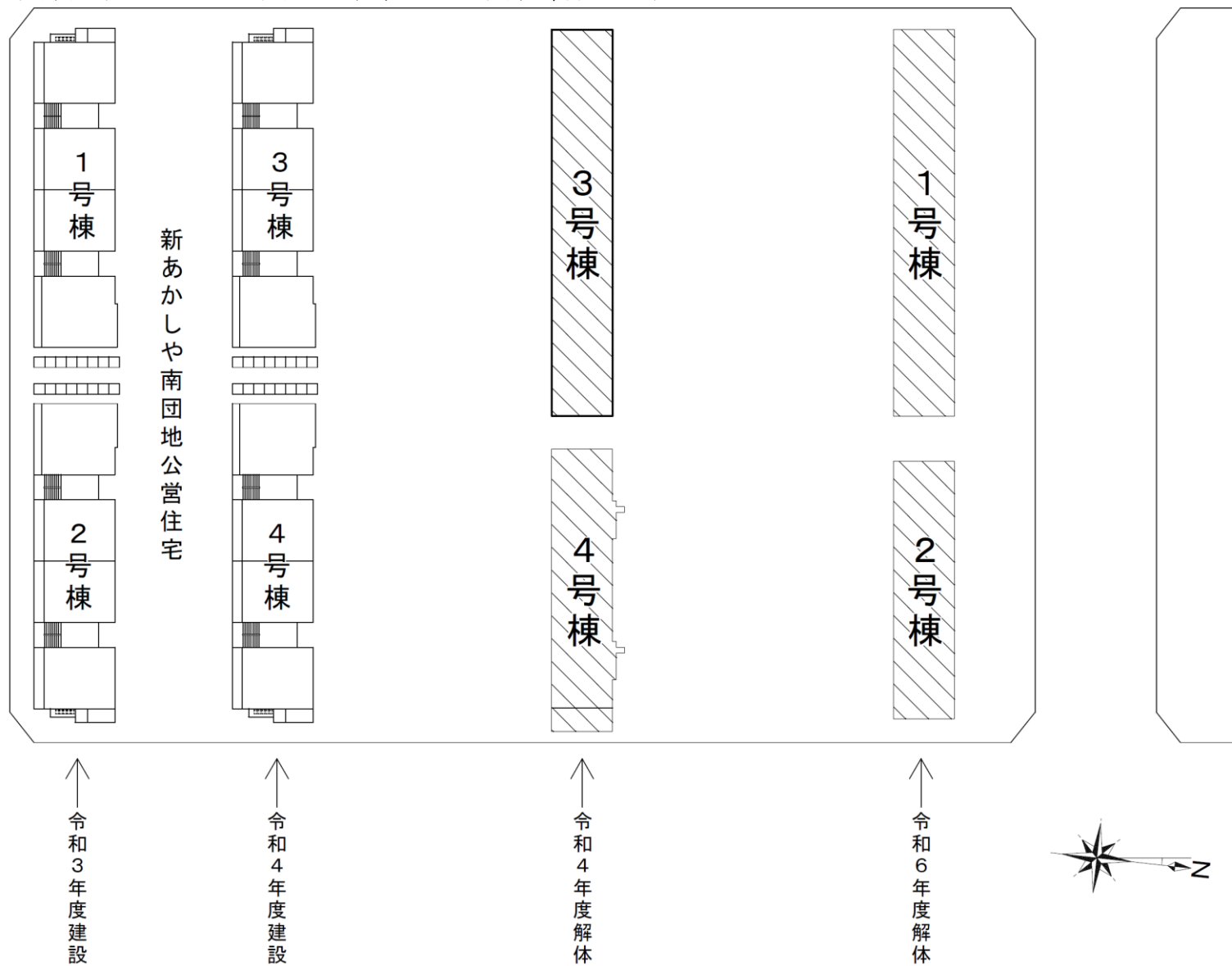
配置図
