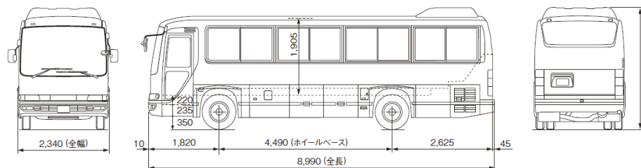
外観図
