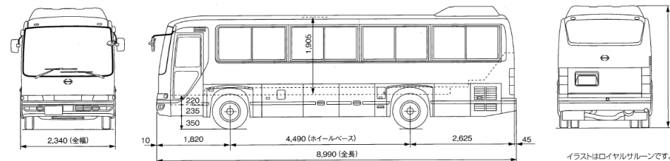
●外観図
