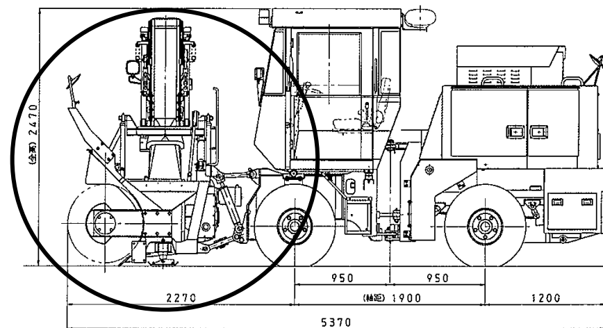
【除雪装置】
