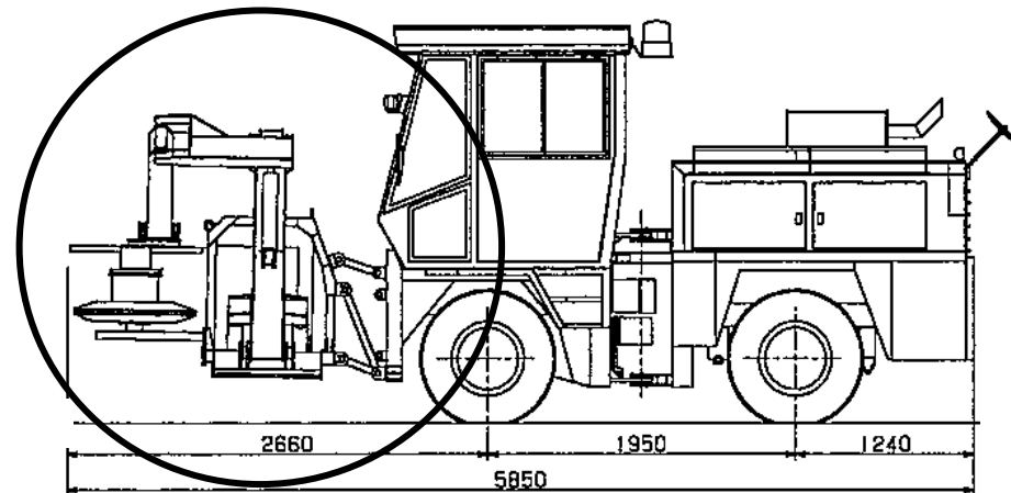
【草刈装置】
