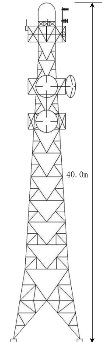
豊岡基地局
