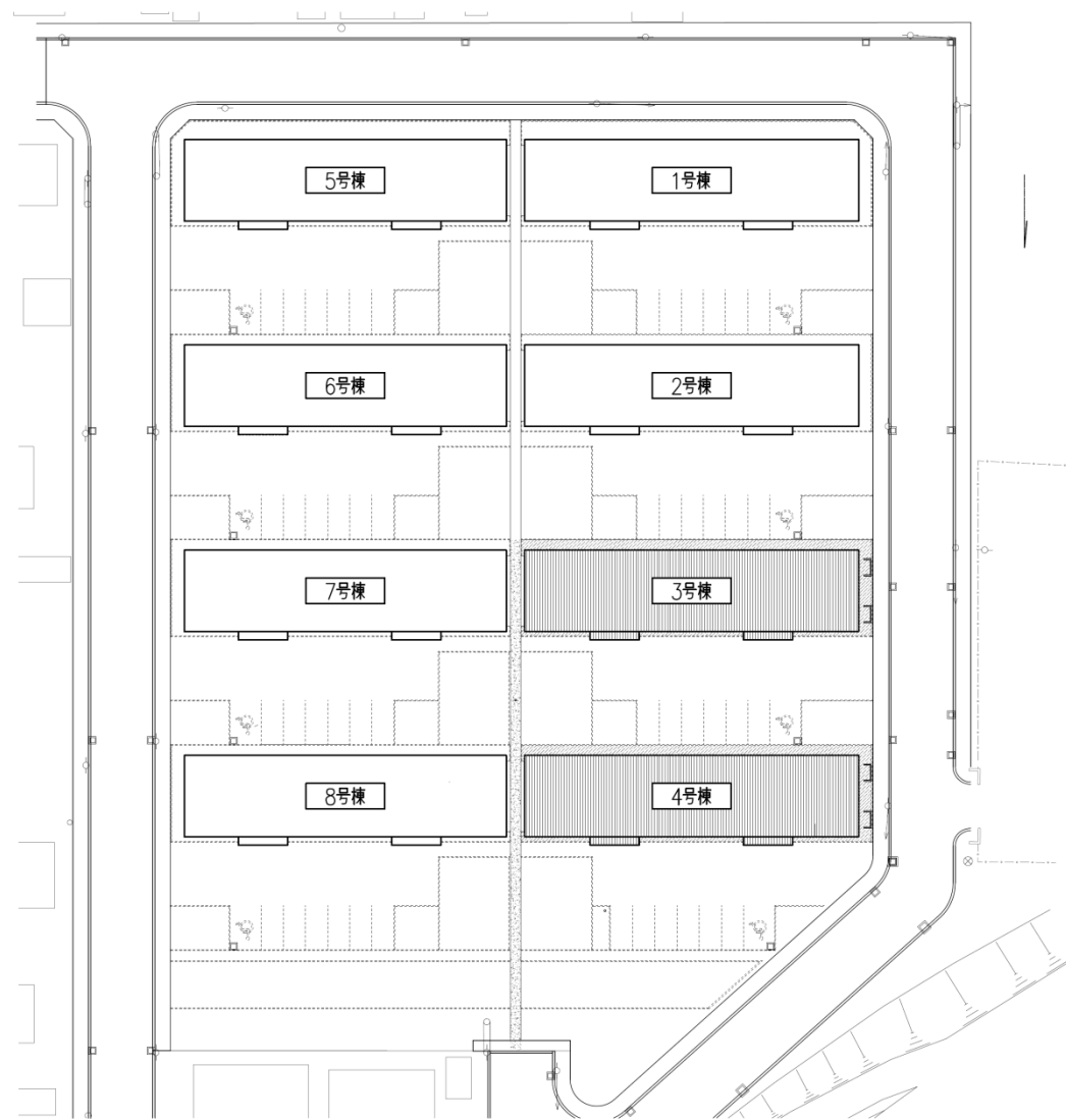
春日東団地公営住宅 配置図
