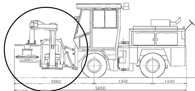
【草刈装置】
