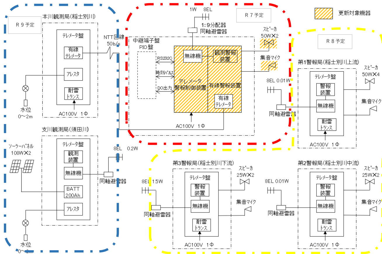
幕別ダム テレメータ・放流警報設備構成図
