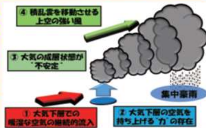
線状降水帯の発生メカニズムの模式図
