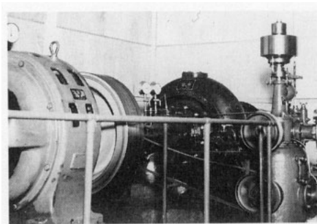
▲忠類村に灯りをともした発電タービン
