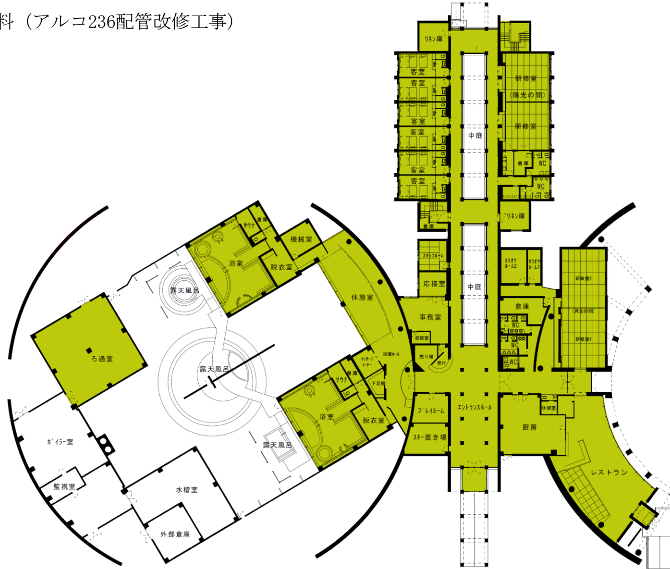
1階平面図
