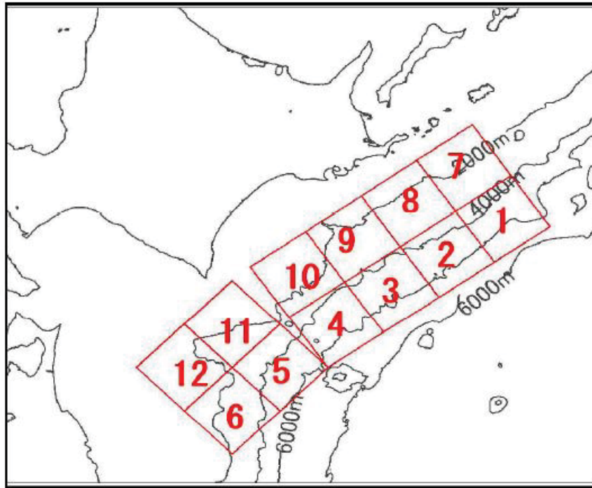
図1-7-2 平成24年度想定地震津波の断層配置図
